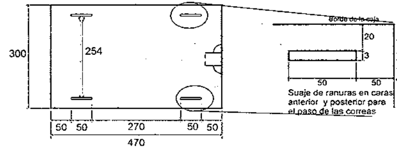
DETALLE DE SUAJES CIRCULARES Y RANURAS PARA ASA Y CORREAS
