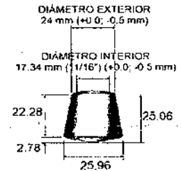
Diám 25.96 mm
