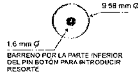
VISTA INFERIOR
