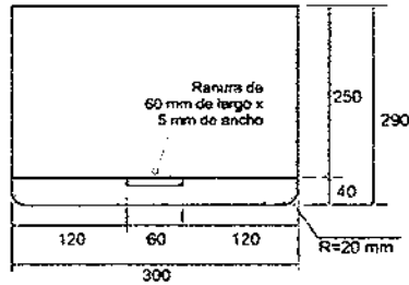
DETALLE DE SUAJES EN TAPAS LATERALES
